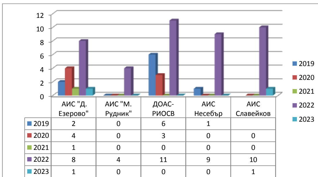
Фиг.2 Брой превишения на СДН на \text{ФПЧ}_{10} в пунктовете за мониторинг ДОАС-РИОСВ, АИС „Долно Езерово“, АИС „Меден Рудник“, АИС „Славейков“, АИС „Несебър“ за периода април-септември на 2019 г., 2020 г., 2021 г., 2022 г. и 2023 г.
